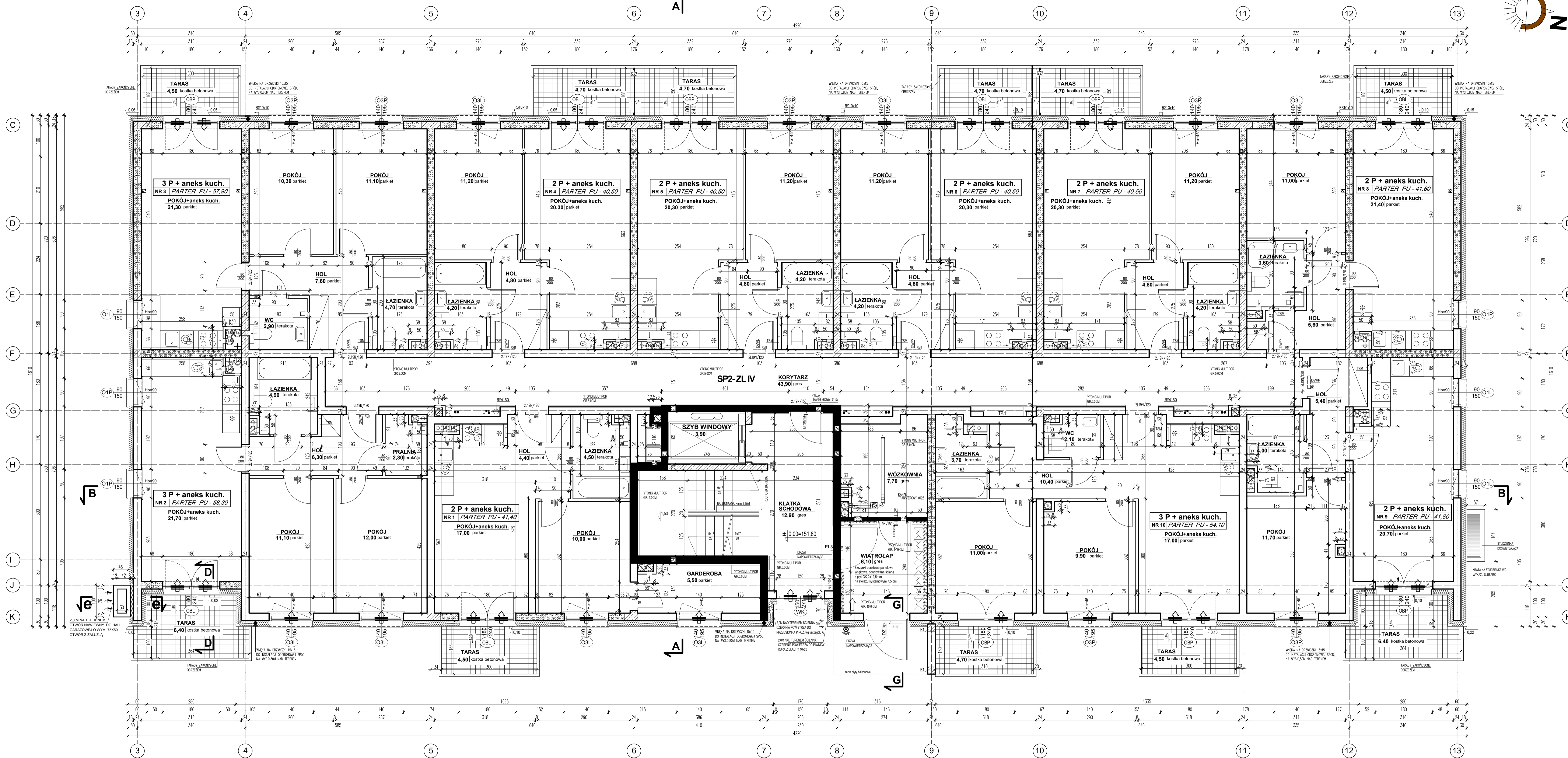
RZUT PARTERU
